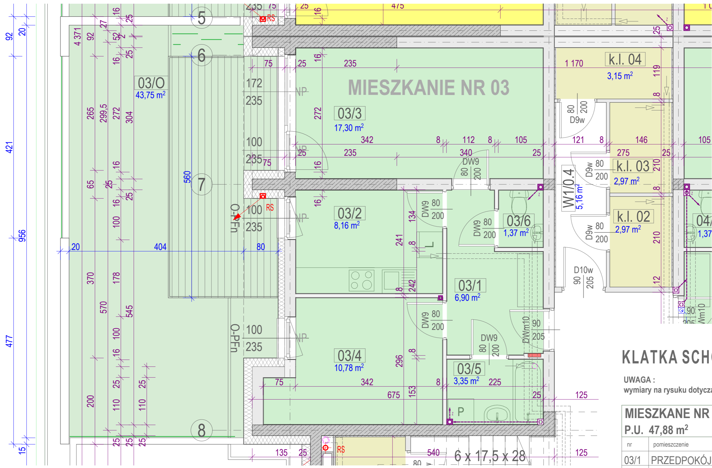
BUDYNEK "A" SKALA 1 : 50
